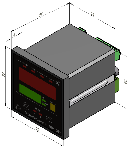
Рис.1. Внешний вид и установочные размеры блока индикации.
